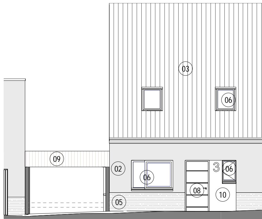
1 ML4 Maison 06 ELEVATION NORD OUEST
