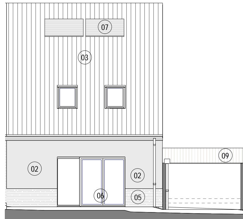
2 ML4 Maison 06 ELEVATION SUD EST
